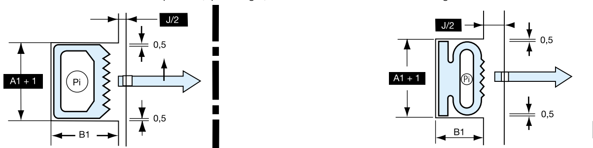
Interne radiale expansie (opstelling II) De werkdruk P_i is 20 tot 30% hoger dan de normale druk.
